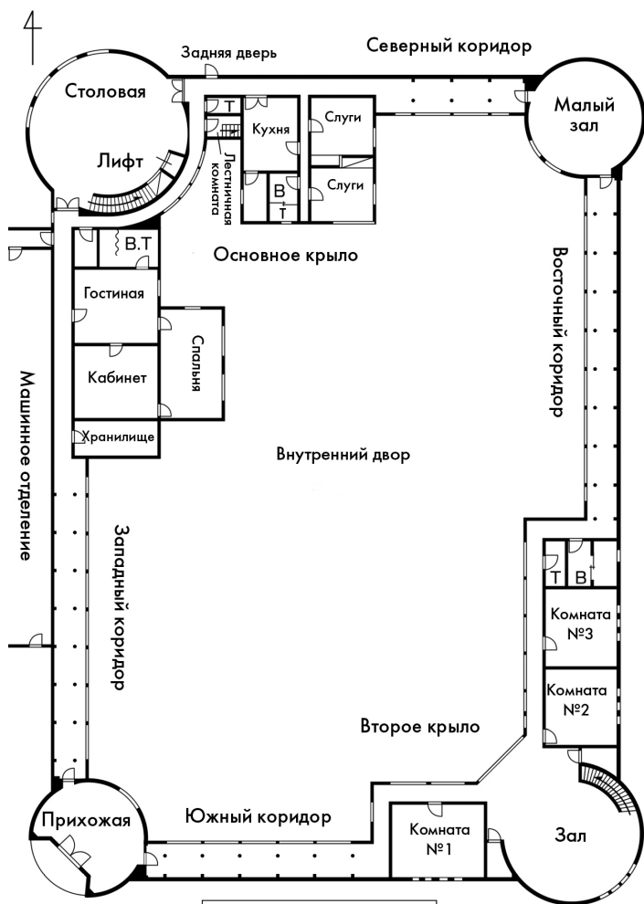
План Дома с водяными колесами, 1-й этаж
