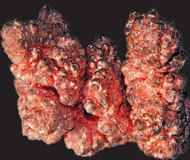
Самородок меди
